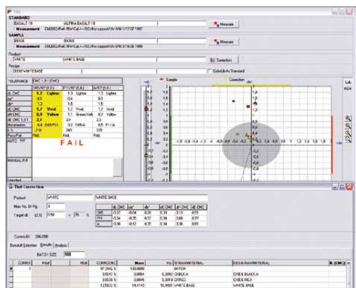
Qualitätskontrolle in der Produktion mit Abtönkorrekturvorschlag
